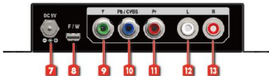
[図 3.2] リアパネルの外観図
